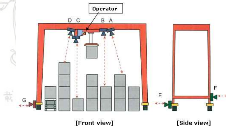
移載機操作示意圖
