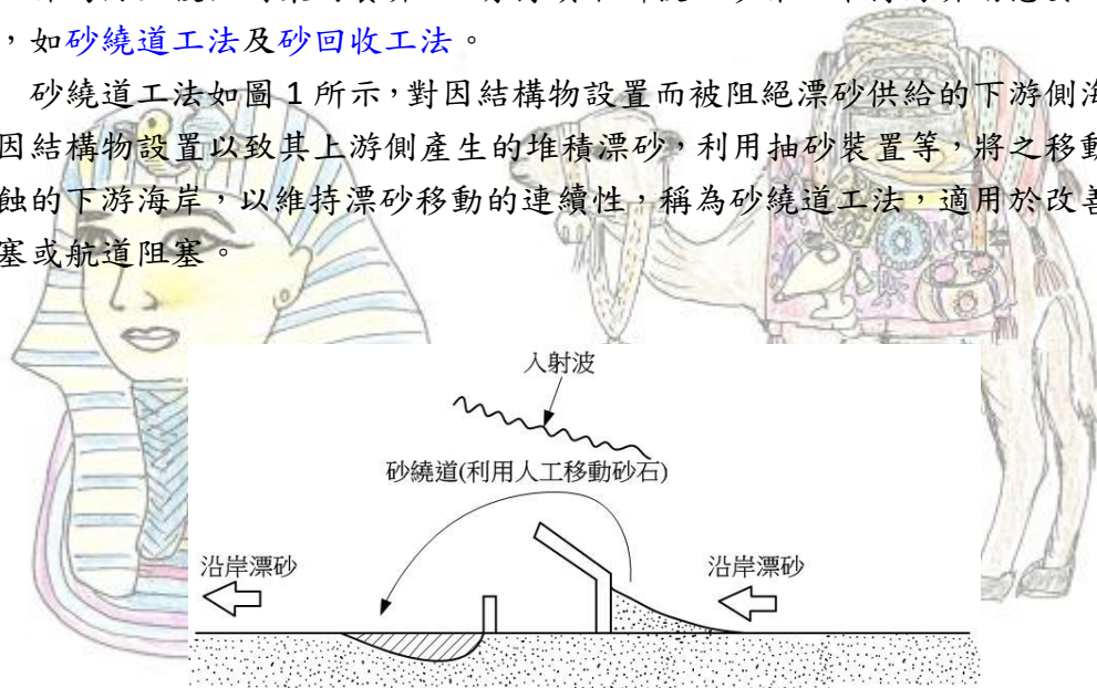
圖 1 砂繞道工法
