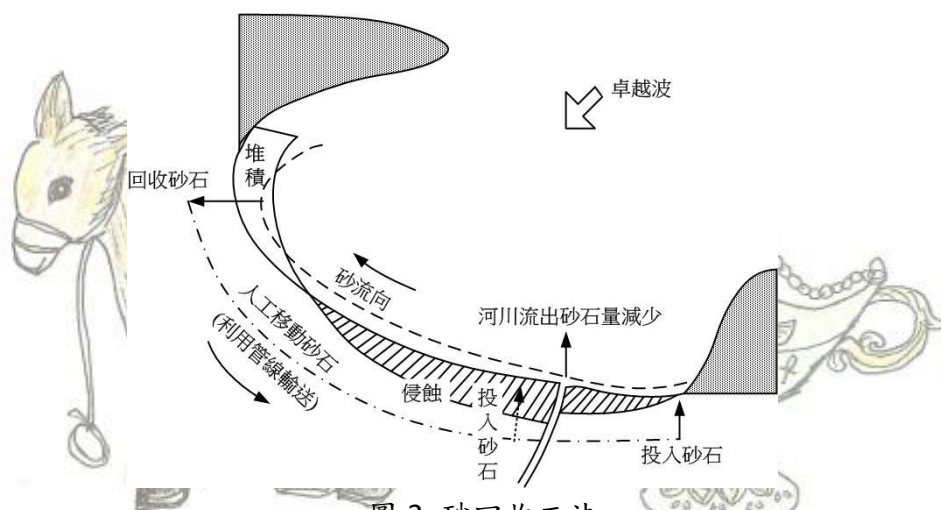
圖 2 砂回收工法
