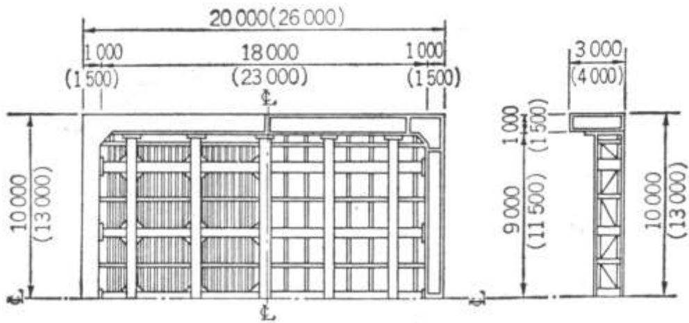
20x20x3m繫浮塢結構圖 ( )為26x26x4m
