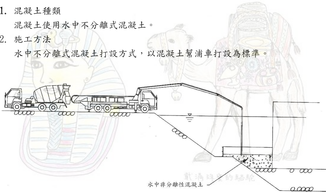
打設概要圖
